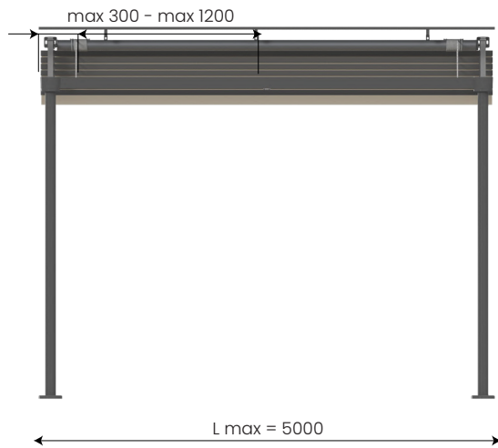
Installazione a 2 colonne Installation on 2 columns
