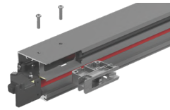
Blocco automatico per tensionamento del telo Automatic locking system for fabric tension
